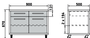
Тумба подкатная
