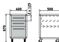
Тумба подкатная
