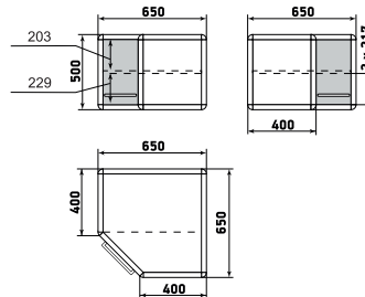
Шкаф навесной
