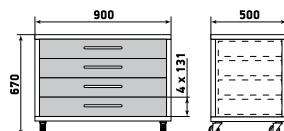
Тумба подкатная
