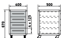
Тумба подкатная
