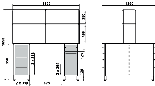
Островной стол
