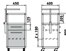
Тумба подкатная
