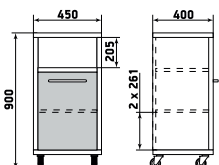
Тумба подкатная
