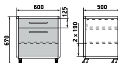
Тумба подкатная
