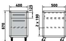
Тумба подкатная
