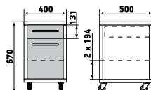
Тумба подкатная
