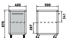
Тумба подкатная
