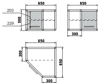
Шкаф навесной
