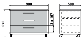
Тумба подкатная
