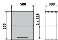
Шкаф навесной
