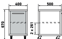
Тумба подкатная
